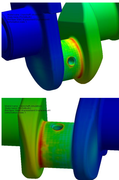
Fig. 9. Zonele de risc cu deplasări maxime în cazul încărcării fusului 1
